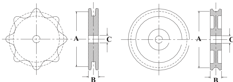
Drive Sprockets
